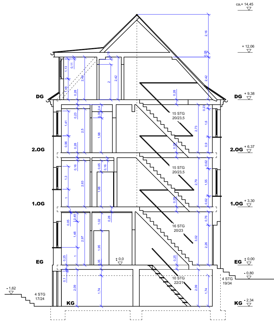
SCHNITT A-A
